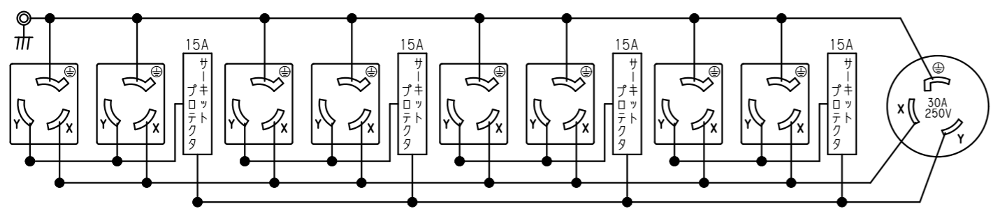
内部配線図
