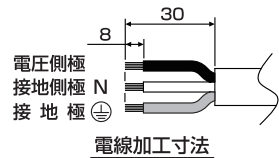
電線加工寸法
