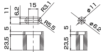
本体取付穴寸法
