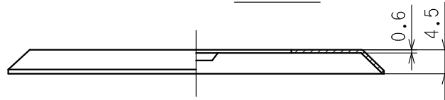
A-O-B断面
