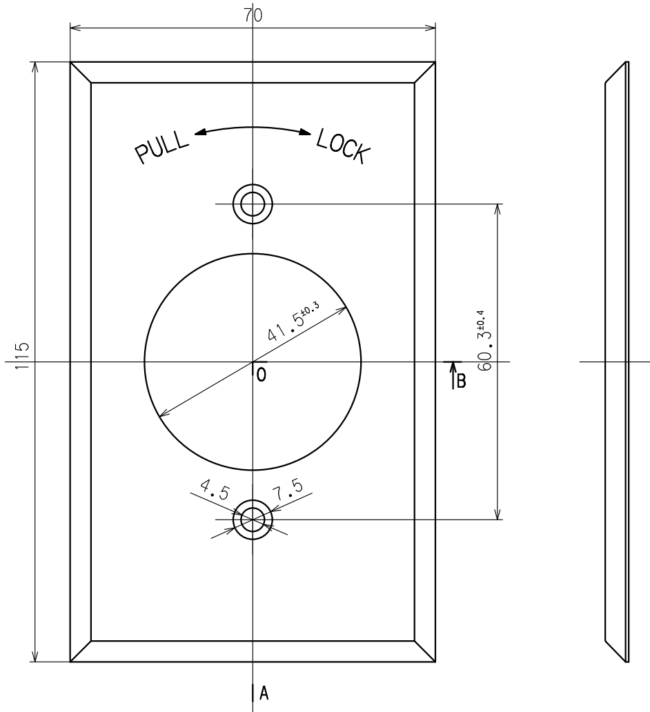
A-O-B断面
