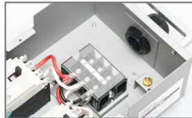
コード口より挿入した14mm 2 電線を端子台に結線して使用します。端子台は透明の絶縁カバー付です。
