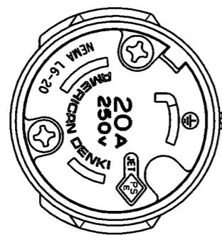
さし込みプラグ正面図
