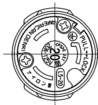
さし込みプラグ正面図
